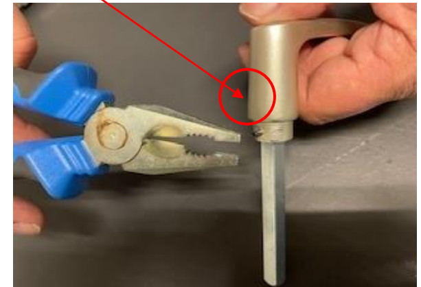
5. Door de indrukking aan de binnenzijde van het stifdeel, komt de borgpin aan de ander zijde naar voren. Tevens breekt door het slaan de lijmverbinding met de stift. Trek de borgpin uit het stifdeel middels de combinatietang
