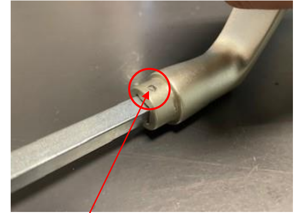
5. Door de indrukking aan de binnenzijde van het stifdeel, komt de borgpin aan de ander zijde naar voren. Tevens breekt door het slaan de lijmverbinding met de stift. Trek de borgpin uit het stifdeel middels de combinatietang
